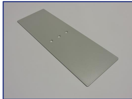
PIEDPLAT 2,7kg 450x150x5mm disponible en blanc ou noir
