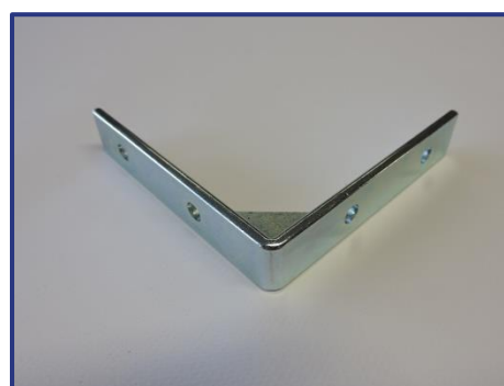
ÉQUERRE 90° HEAVYDUTY équerre pour joindre profilé PL78 et le profilé PL78 ANGLE 90° incl platines de fixation M6 + vis
