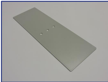
PIEDPLAT 1,6kg 450x150x3mm disponible en blanc ou noir
