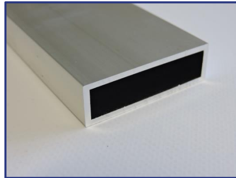
SX 50 raidisseur 50x15x2mm
