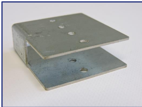
FIX 50 fixation raidisseur SX 50
