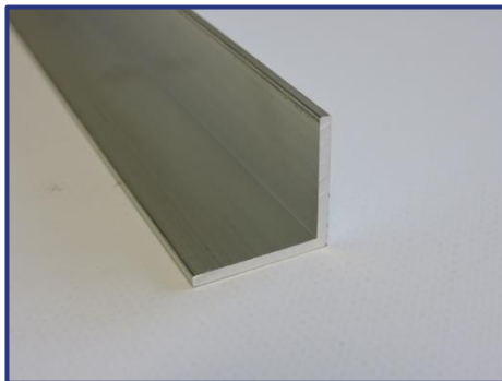
L20 Cornière alu brut ou laquée blanc 25x25mm longueur 6m
